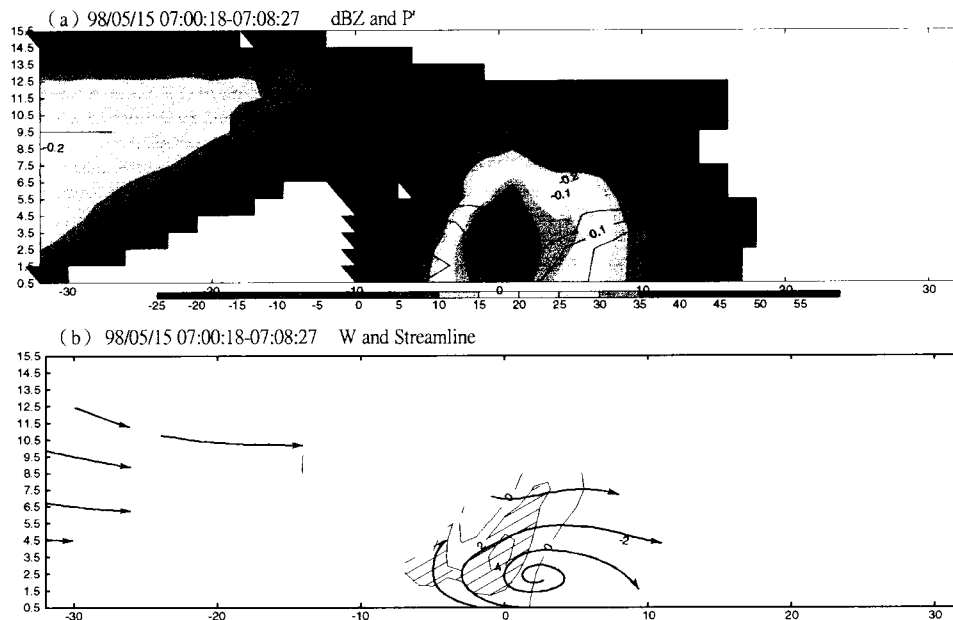
圖五：1998年5月15日0700Z垂直於線狀對流系統之垂直剖面 (a) 擾動壓力場疊加上回波場 (b) 相對系統運動之流線場疊加上垂直速度場，實線為正值，虛線為負值。
