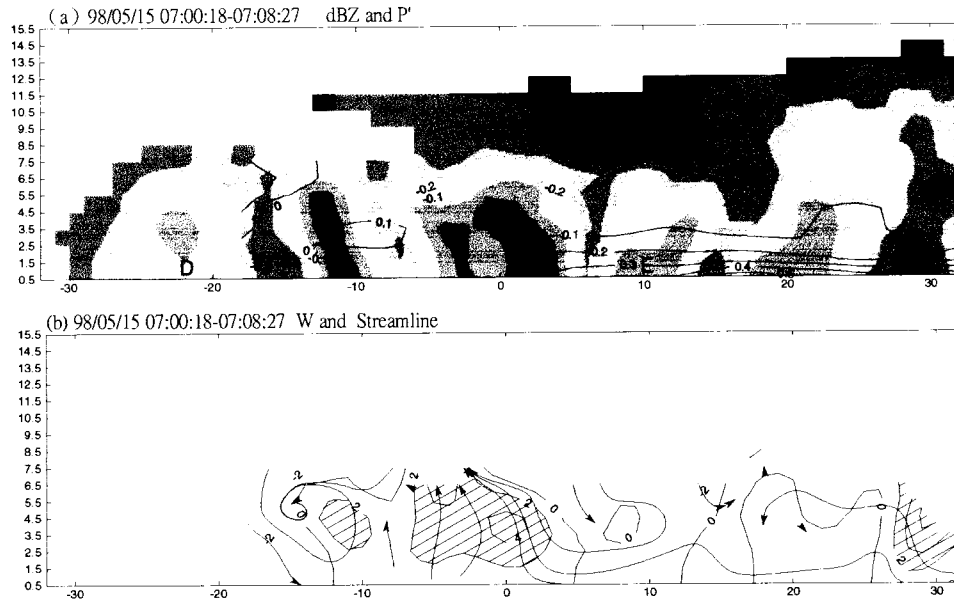
圖四：1998年5月15日0700Z之平行於對流系統之垂直剖面，(a) 等值線為擾動壓力場疊加回波場，(b) 相對系統運動之流線疊加垂直速度場，實線為正值，虛線為負值，垂直速度大於2m/s以斜線表區。
